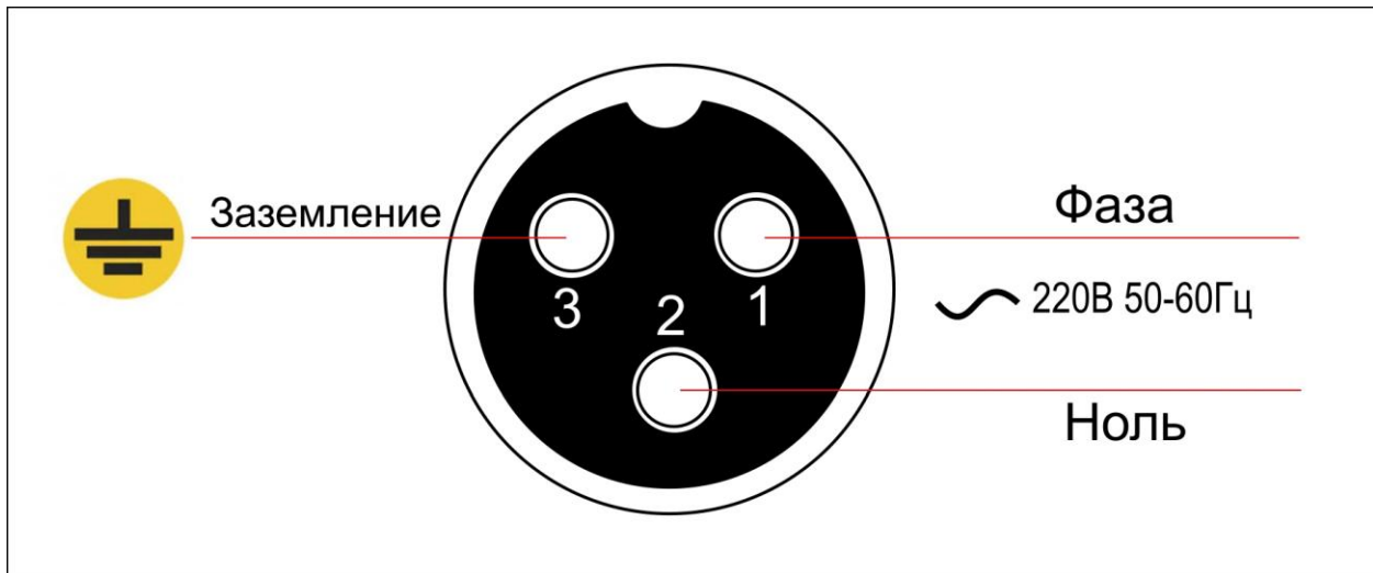
Рисунок 2.1. Маркировка разъёма «Питание»
